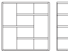
art. SUR 170 L/W 170 H 175 P/D 40 W 66,9" H 68,9" D 15,7"
